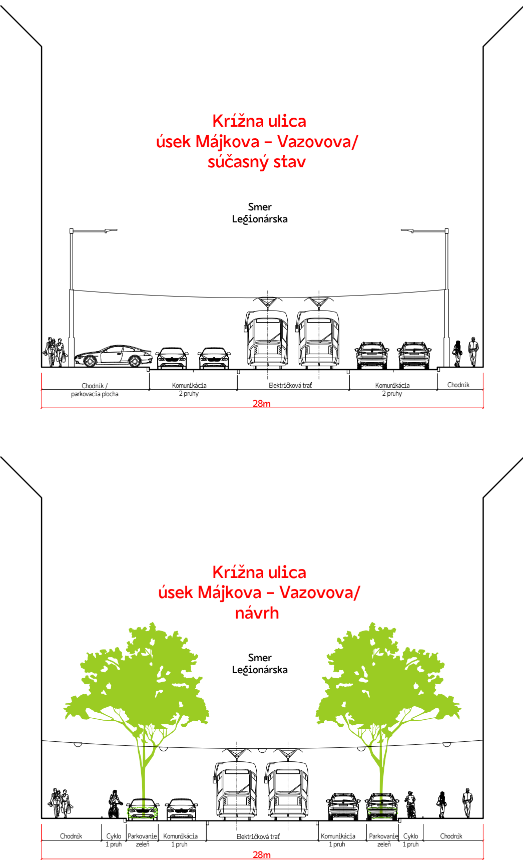
Návrh profilu Krížnej ulice v prípravnej fáze projektu
