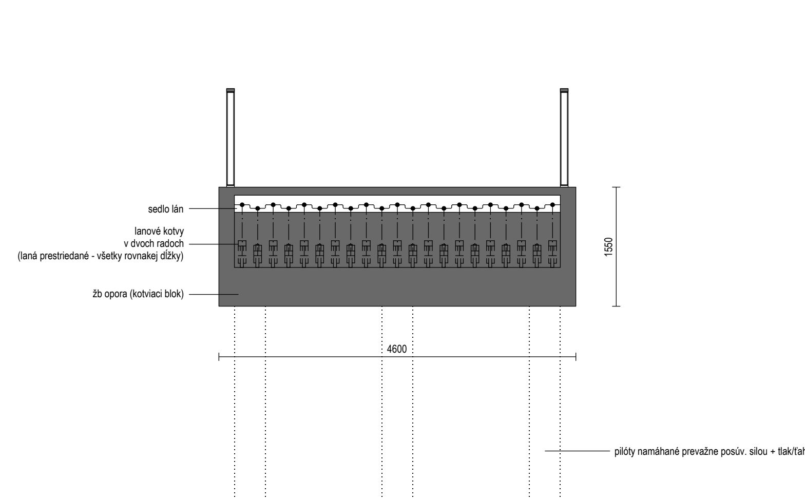
nad oporou 2 1:50
