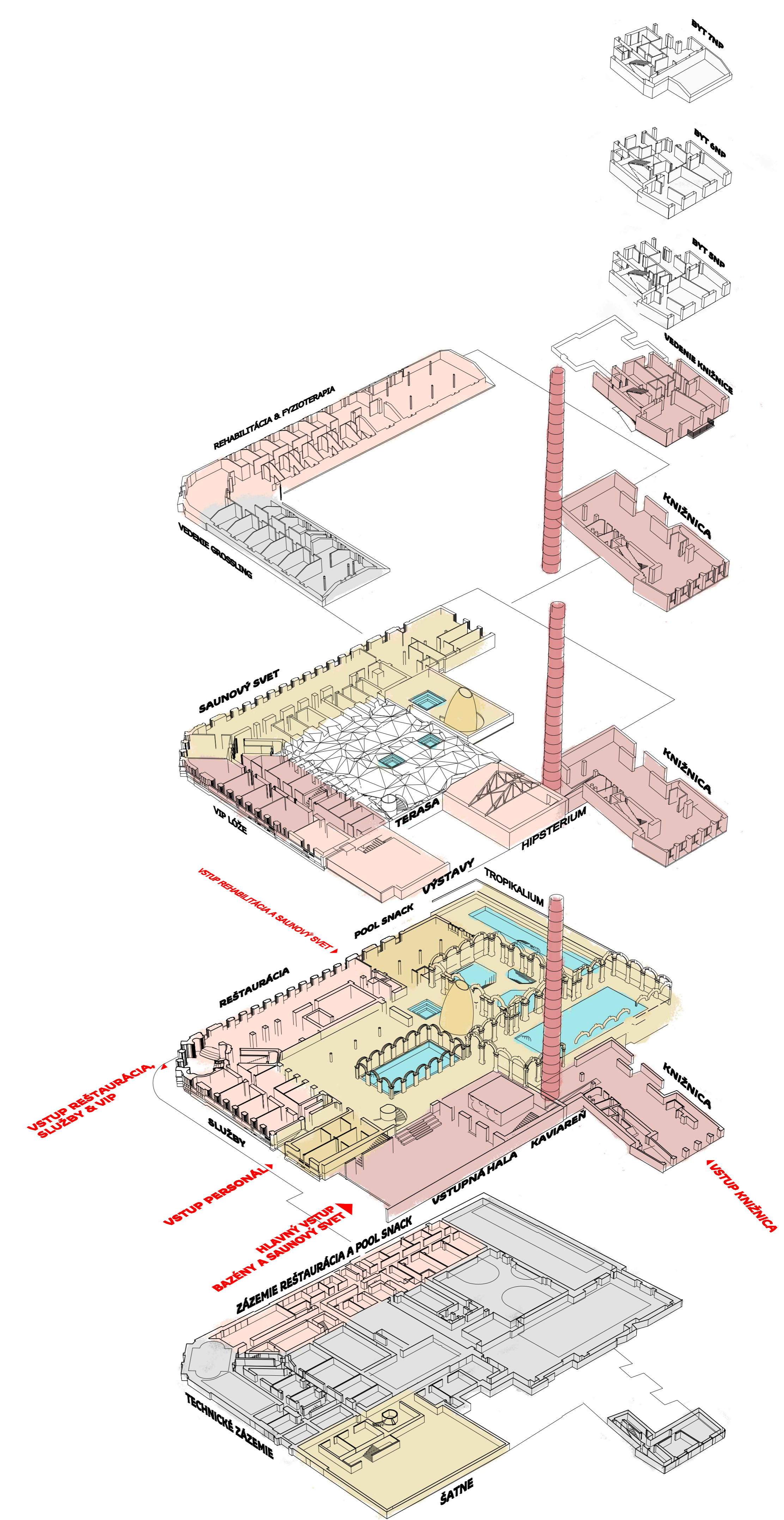
VSTUPNÁ HALA
